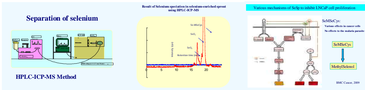
HPLC-ICP-MS法
